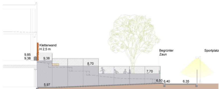
Schnitt B
