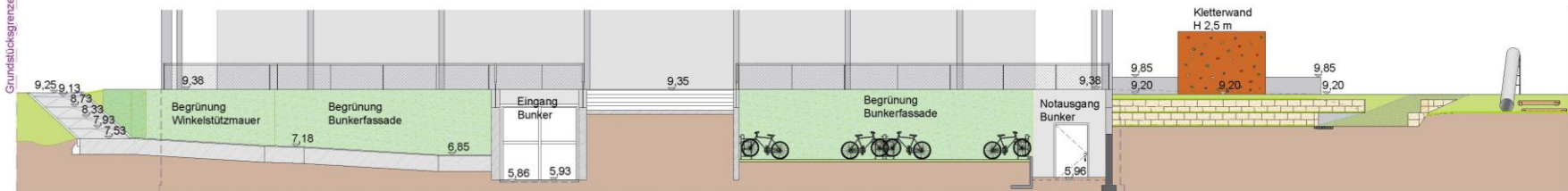
Schnitt C
