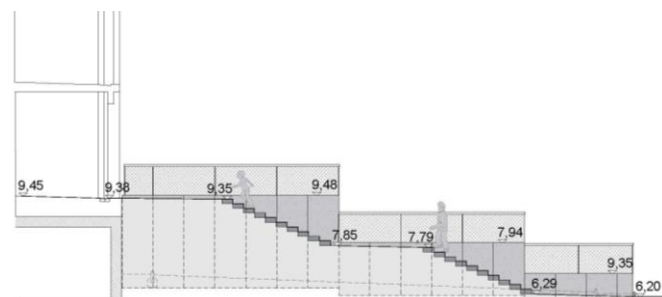
Schnitt D
