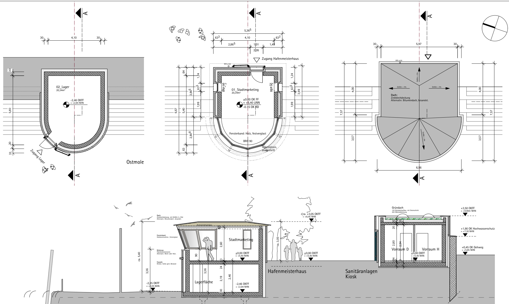
Grundrisse und Schnitte - ohne Maßstab
