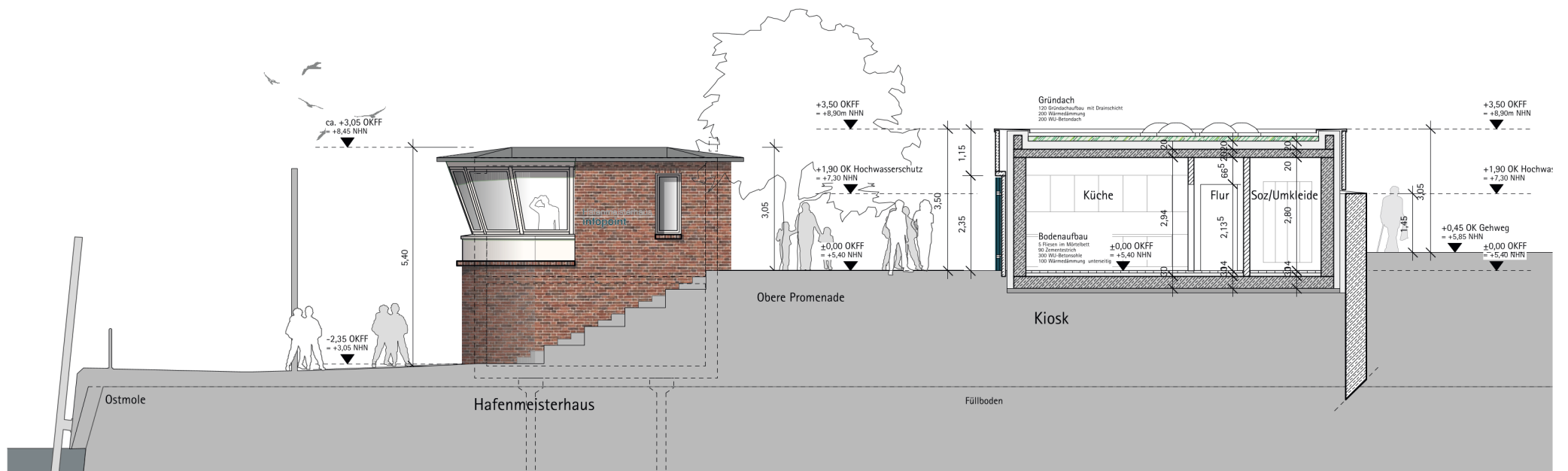
Schnitte - ohne Maßstab
