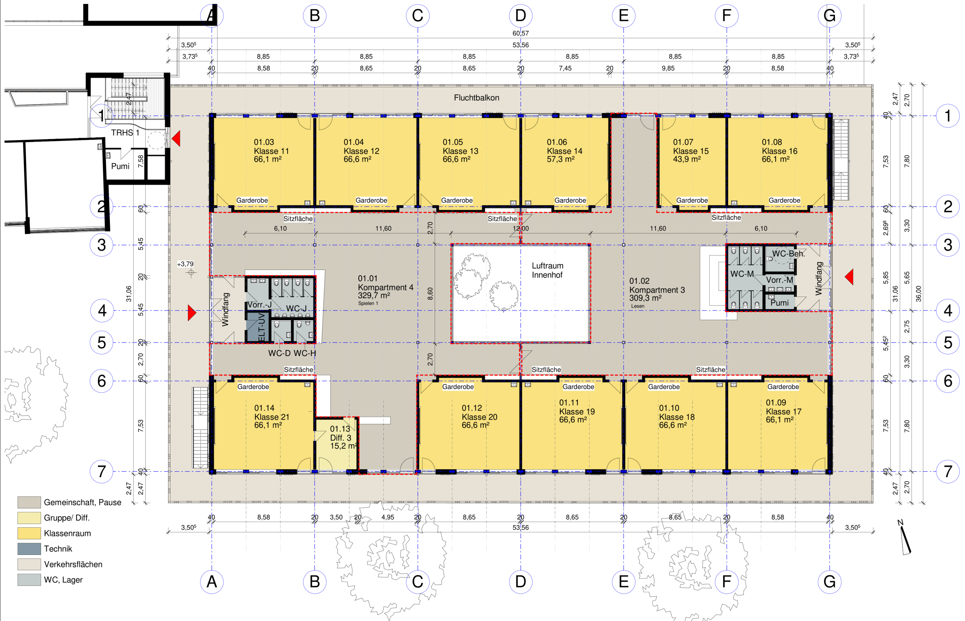
01 1. Obergeschoss M: 1 : 200
