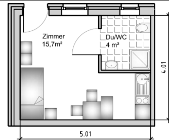
Grundriss einer Wohneinheit M 1:100
